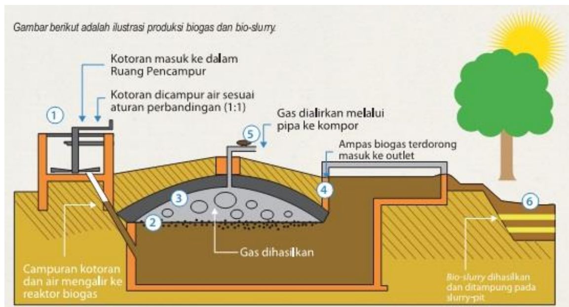
Gambar 2. Ilustrasi teknologi biogas 5
